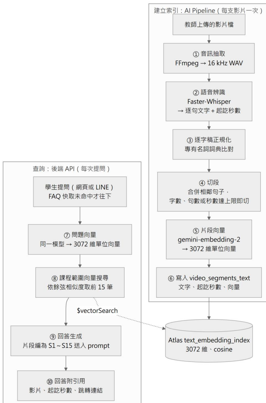
圖 7-2-6 向量化與檢索流程圖
