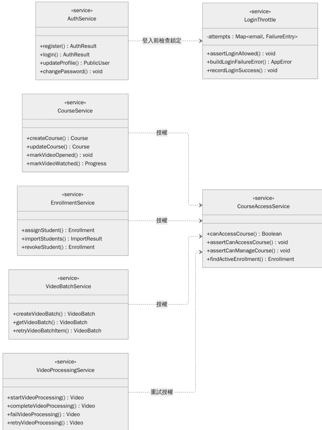
圖 6-2-1a 帳號課程與影片服務設計類別圖
