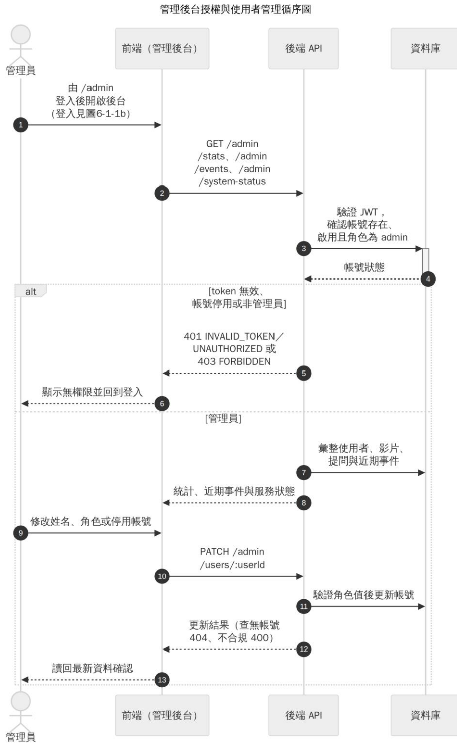
圖 6-1-9a 管理後台授權與使用者管理循序圖
