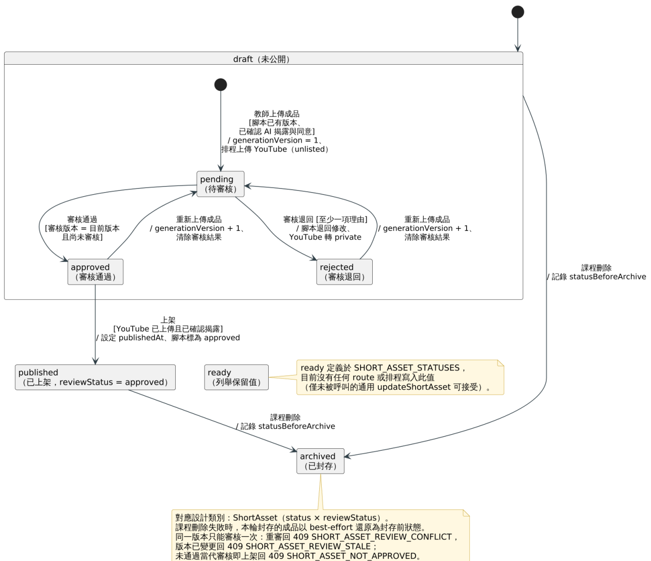
圖 7-4-8 短影音成品狀態機圖
