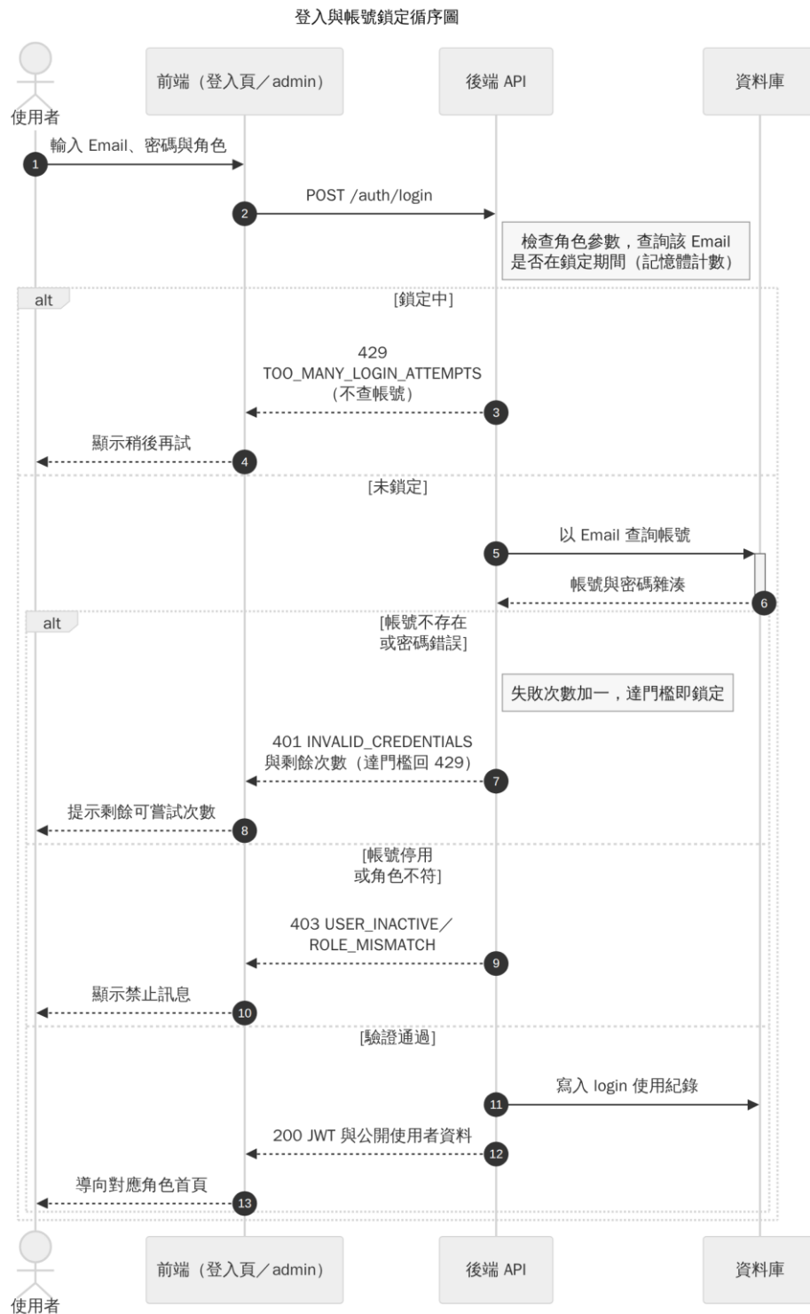
圖 6-1-1b 登入與帳號鎖定循序圖
