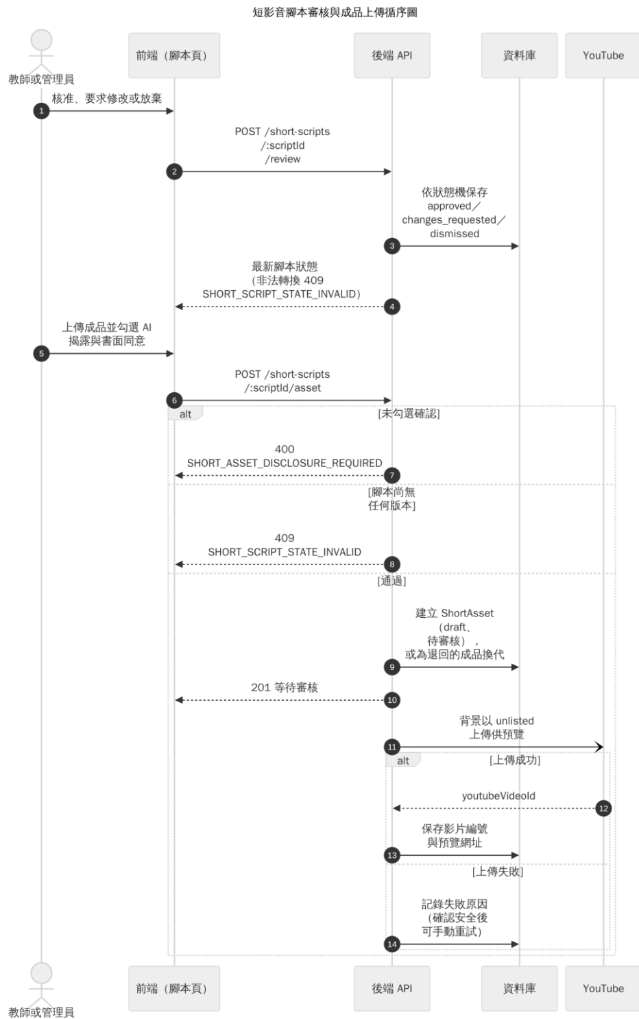
圖 6-1-8b 短影音脚本審核與成品上傳循序圖
