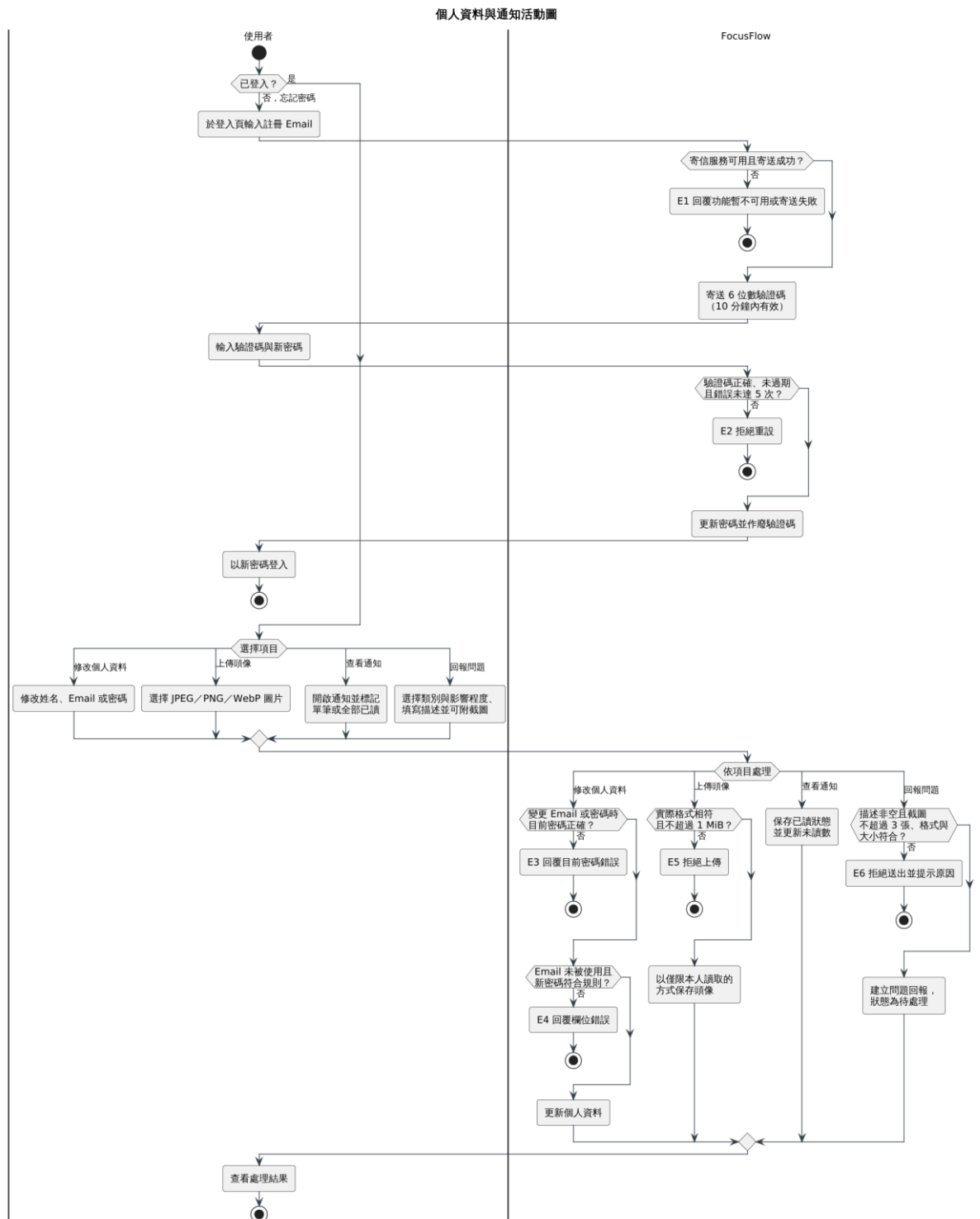
圖 5-3-6 個人資料與通知活動圖
