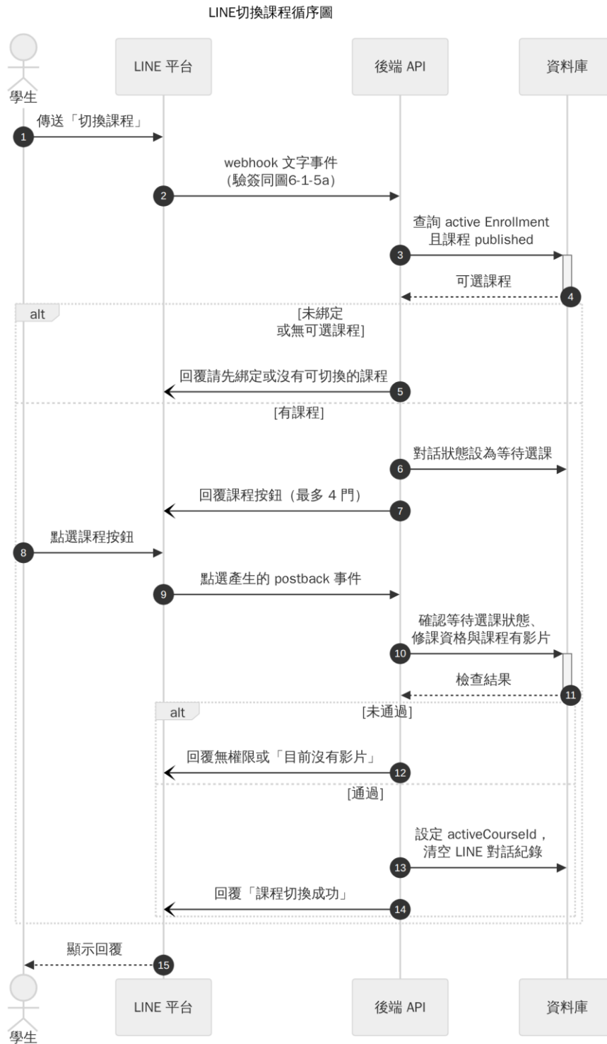
圖 6-1-5b LINE 切換課程循序圖
