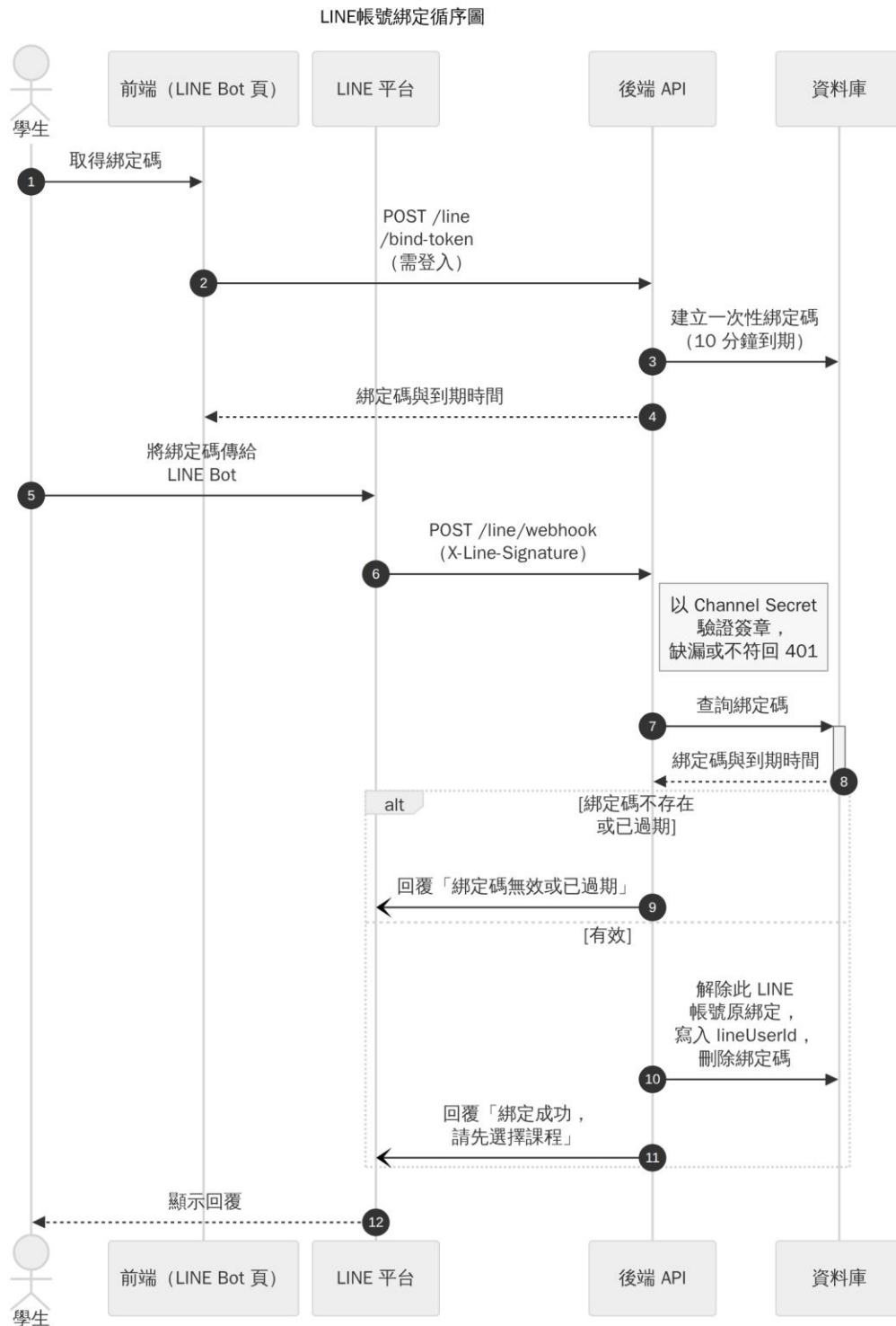
圖 6-1-5a LINE 帳號綁定循序圖
