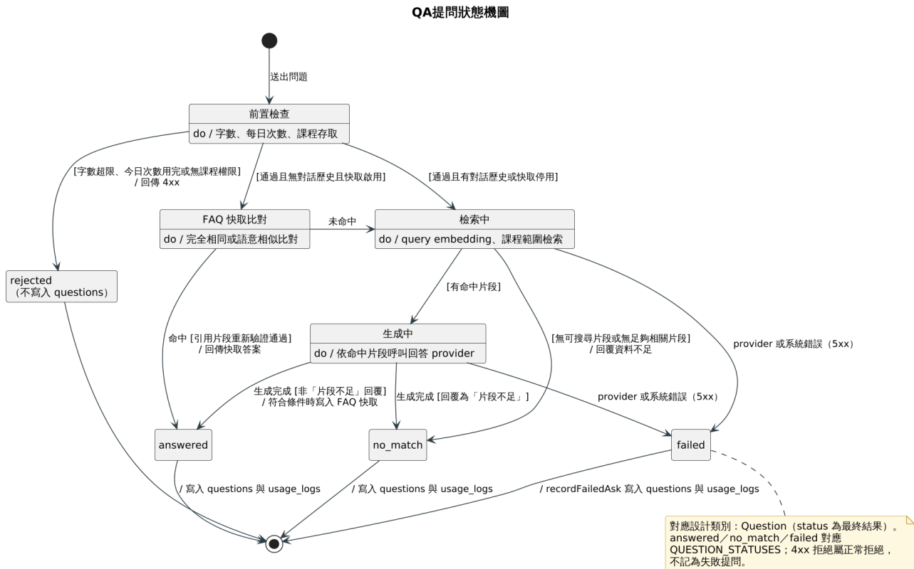
圖 7-4-4 QA 提問狀態機圖
