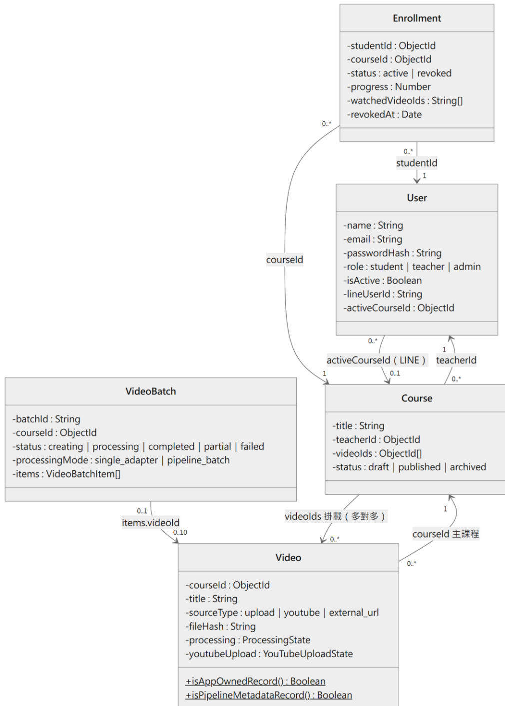
圖 6-2-1b 帳號課程與影片資料設計類別圖
