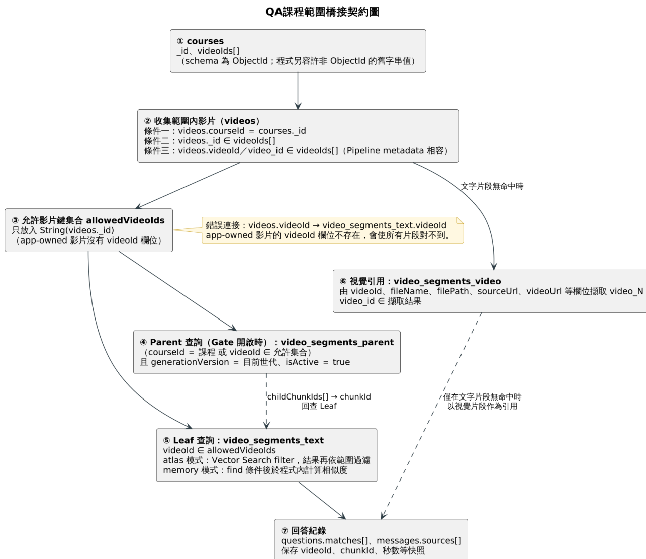
圖 8-1-6 QA 課程範圍橋接契約圖
