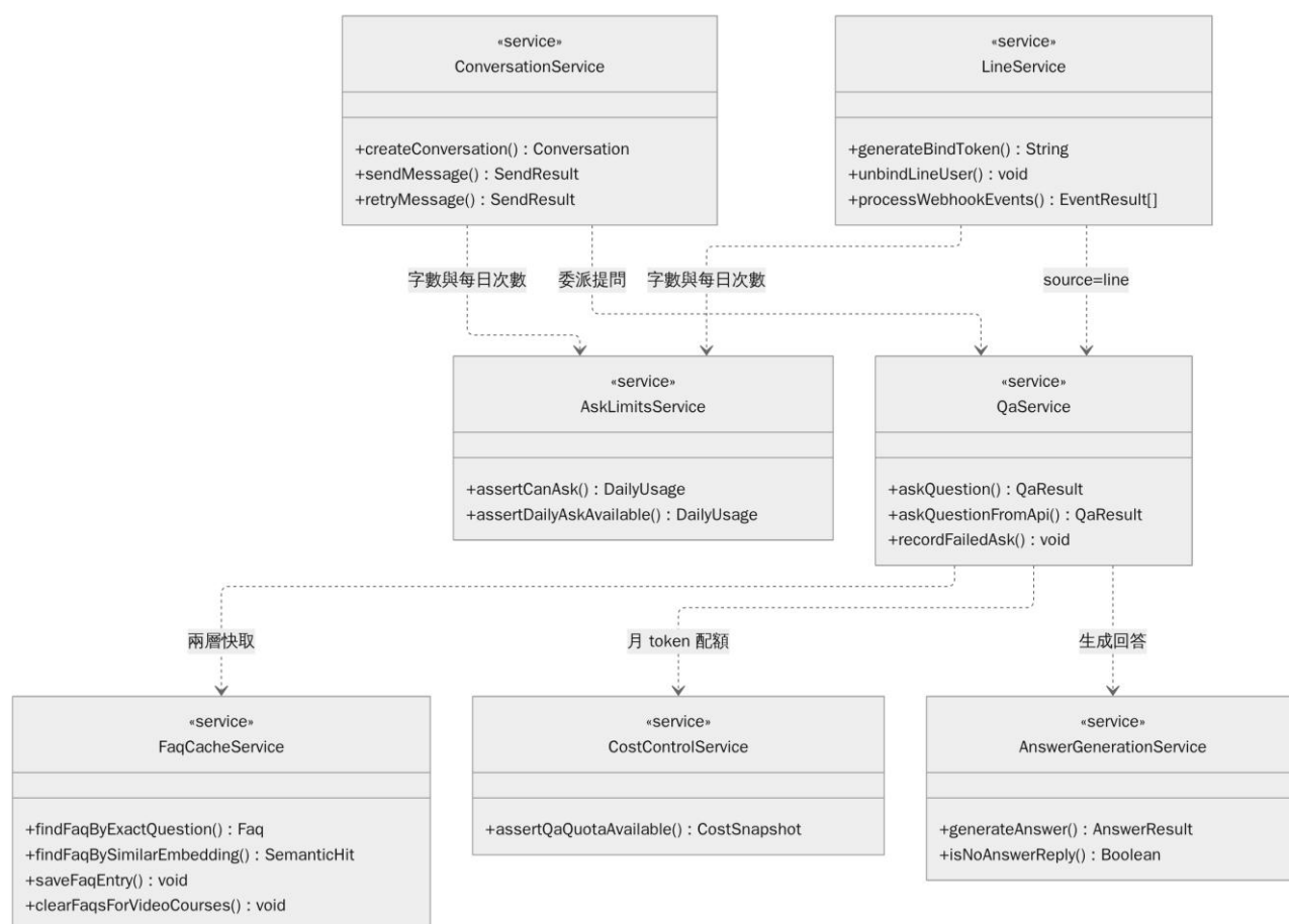
圖 6-2-2a 問答與對話服務設計類別圖
