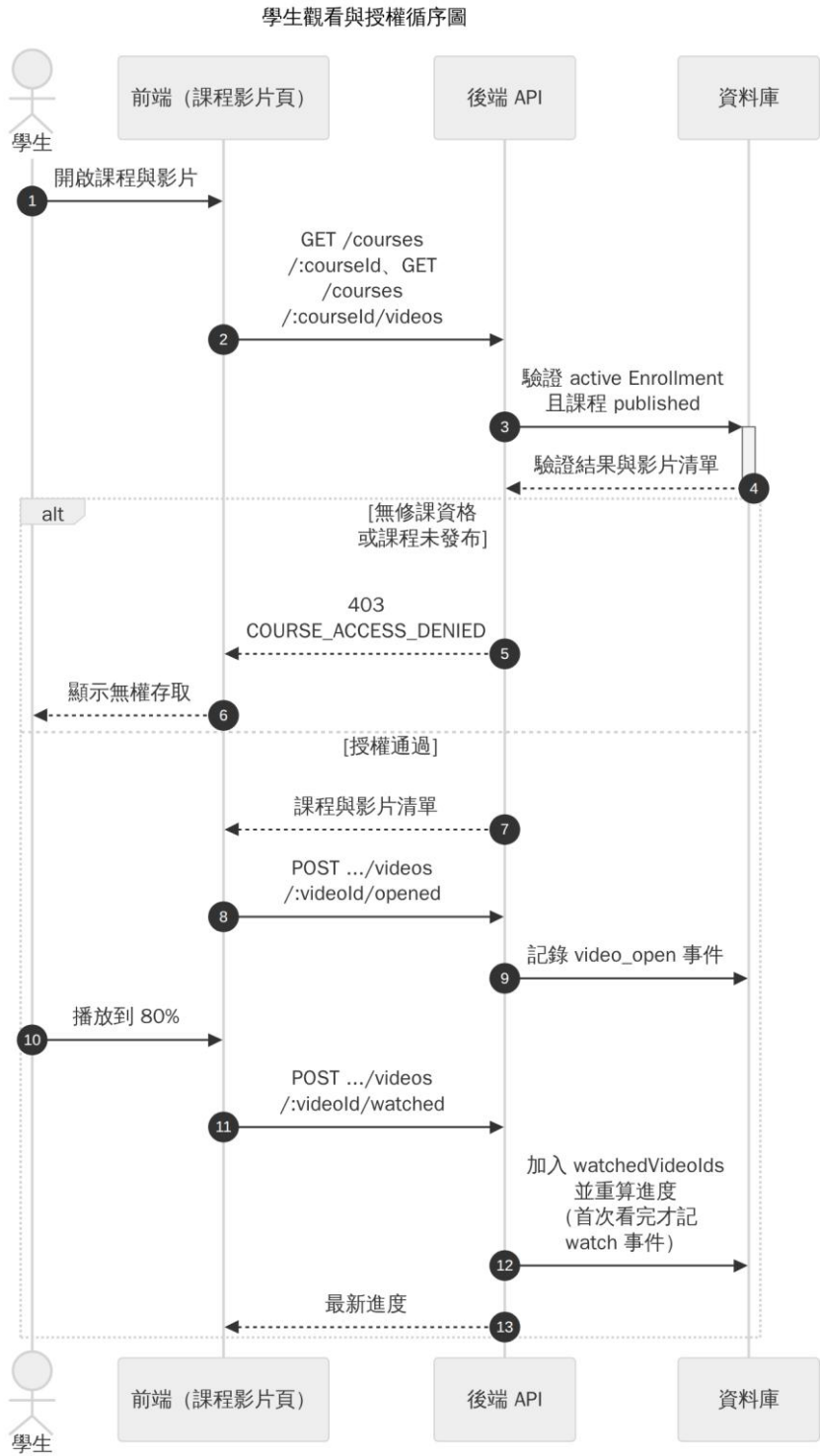
圖 6-1-4a 學生觀看與授權循序圖
