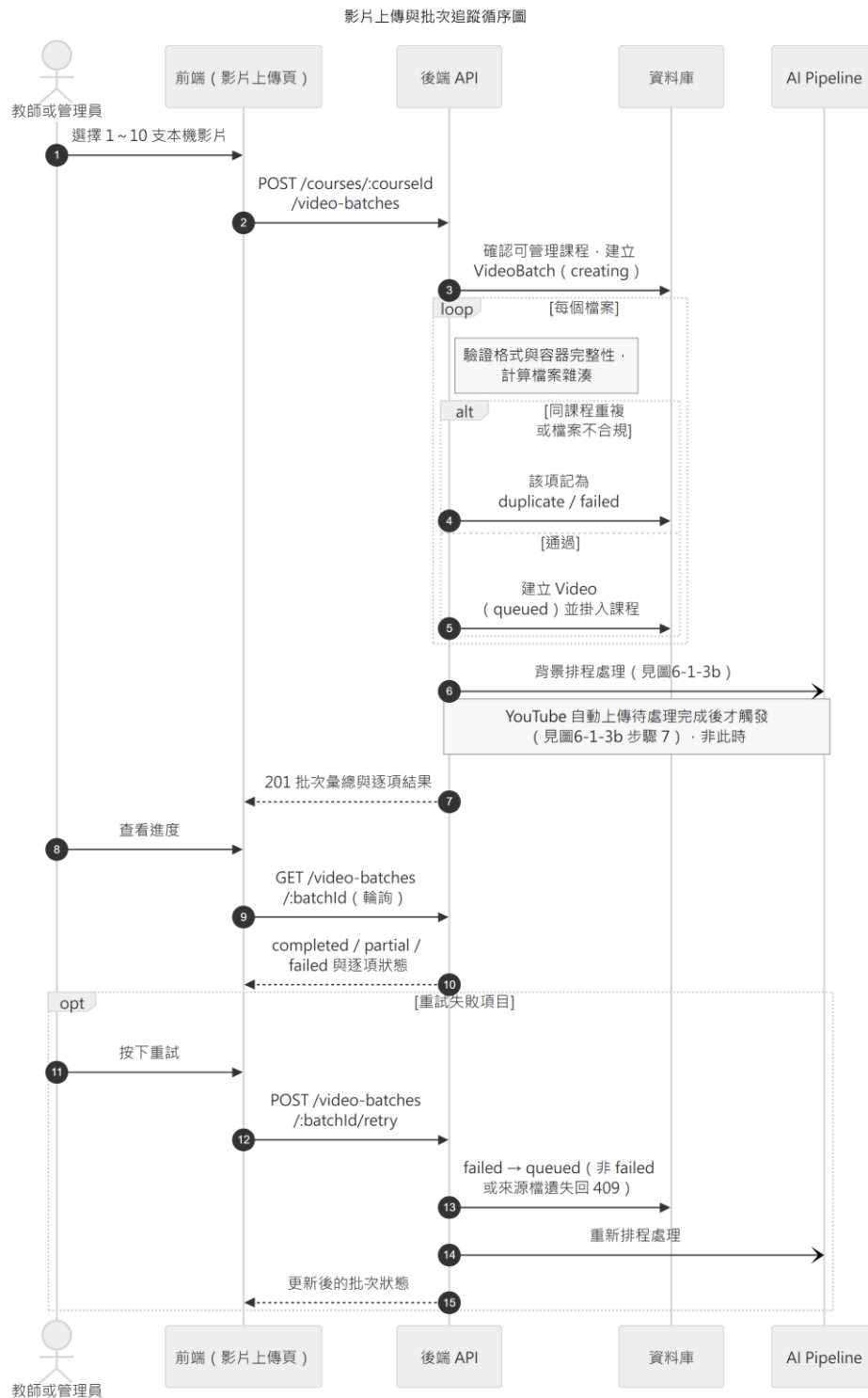
圖 6-1-3a 影片上傳與批次追蹤循序圖
