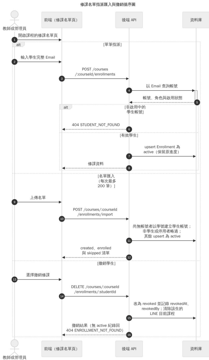
圖 6-1-2b 修課名單指派、匯入與撤銷循序圖
