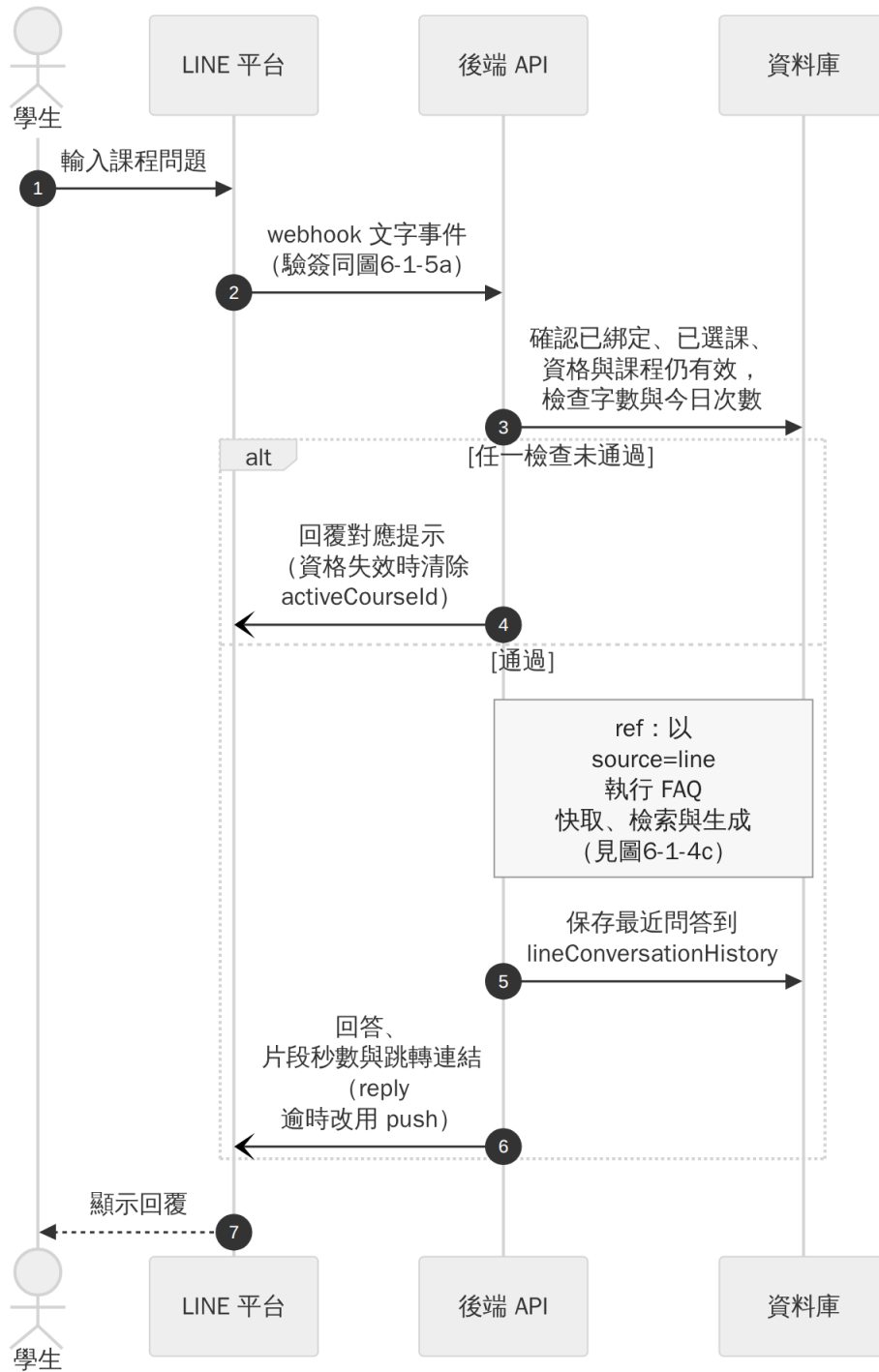
圖 6-1-5c LINE 課程提問循序圖
