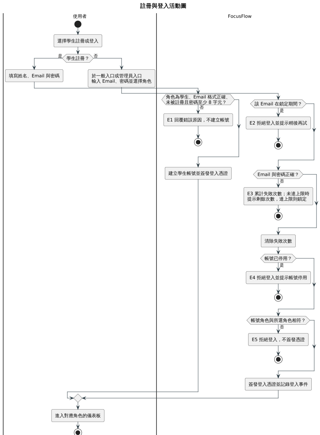
圖 5-3-1 註冊與登入活動圖
